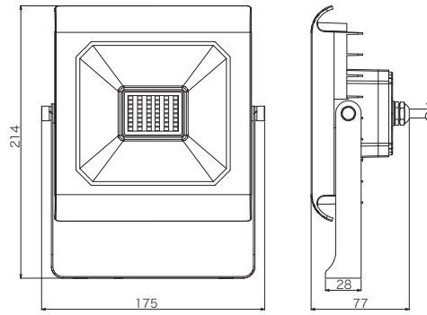
取付部寸法
