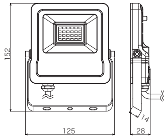
取付部寸法
