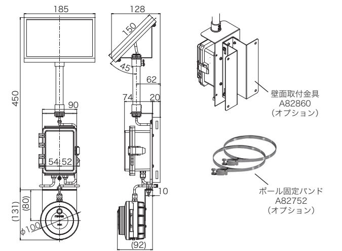
寸法図 (単位 : mm)
