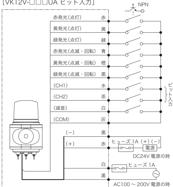
[VK12V-□□□UA ビット入力]
