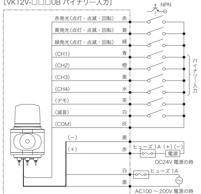
[VK12V-□□□UB バイナリー入力]
