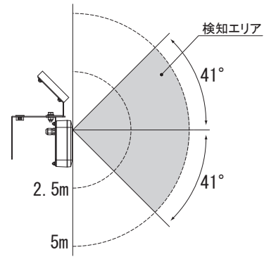
【側面図】・・・製品を横から見たところ
