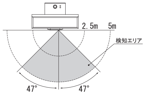
【平面図】・・・製品を上から見たところ
