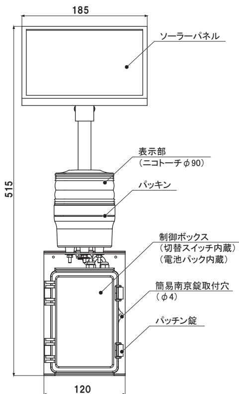
【正面図】
