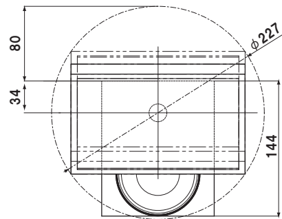
【上面図】
