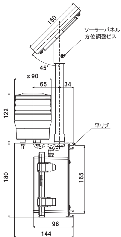
【側面図】
