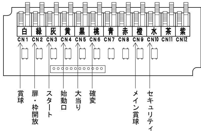
外部接続端子（接点）
